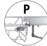
Hammer Tischverlängerung mit Einhebel-Klemmsystem, Breite 150 mm, Länge 400 mm, massiver Grauguss, passend für Hammer Maschinentypen
