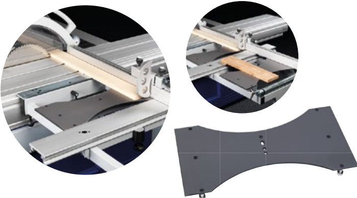
Für 1300 mm und „X-Roll“ 1 Stück, nachrüstbar auf jedem Felder Ausleger 1300 mm mit Werkstückrolle und Format4 Ausleger „X-Roll“
